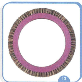
(Artos) \phi 205 \times \phi 145 \times 17
